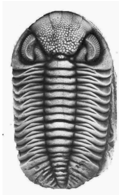
Trilobite
